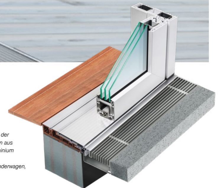
Abb.: Einbausituation schematisch HST 82 mit barrierefreier Schwelle und Bodenanschlussprofilen
