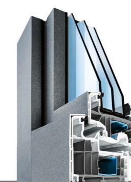
PAST 92 Kunststoff mit Alu-Vorsatzschale 92 mm Bautiefe U_w bis 0,67 W/m 2 K
