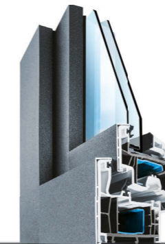
PAST 76 AluColor Kunststoff mit Alu-Vorsatzschale 76 mm Bautiefe U_w bis 0,69 W/m 2 K
